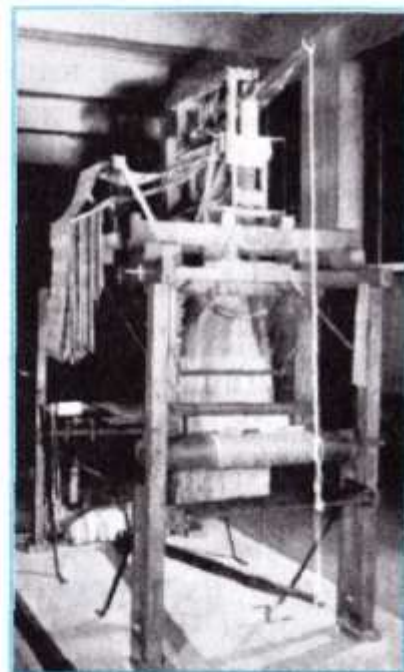
Ткацкий станок Жаккара
